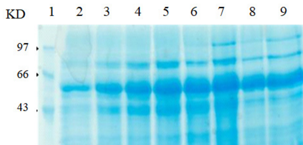
Fig. 2. Expression level analysis of the MDS I in the 5-liter fermentation culture supernatant at different time points by SDS-PAGE, molecular marker (lane 1), 12 h (lane 2), 24 h (lane 3), 48 h (lane 4), 60 h (lane 5), 72 h (lane 6), 84 h (lane 7), 96 h (lane 8), 108 h (lane 9).
